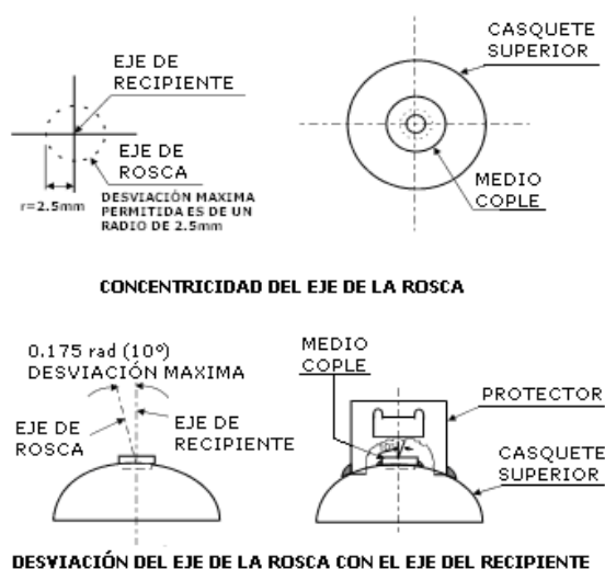
Figura 6.5 Concentricidad y desviación del medio cople con el recipiente
