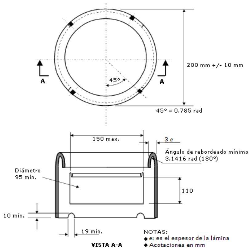
Figura 6.6 Cuello protector
