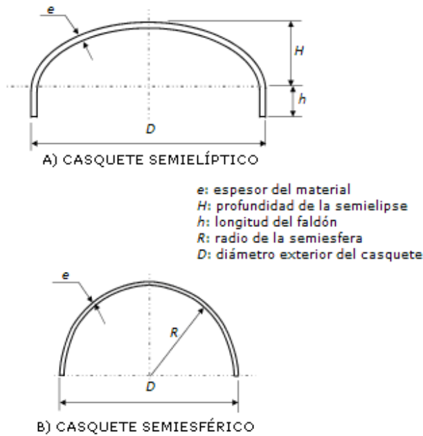
Figura 6.3 Formas de casquete
