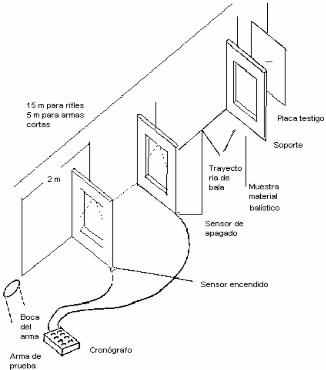
Figura 2.- Esquema ilustrativo para determinar el nivel de resistencia a los impactos de bala.
