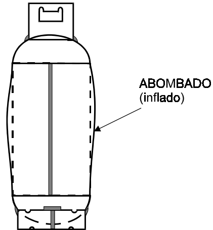
Figura B: Recipiente portátil con abombamiento
